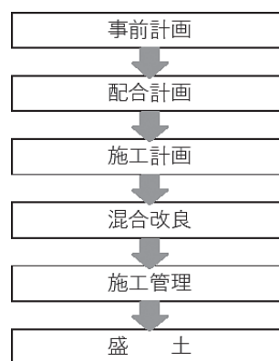
図-2 土砂混合工の流れ
