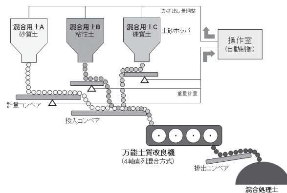
図-4 万能土質改良システムのフロー
