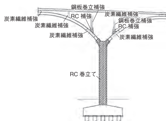
図－2 側面図
