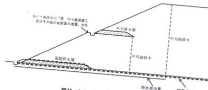
図 V-2-1 盛土の排水施設の概要図
